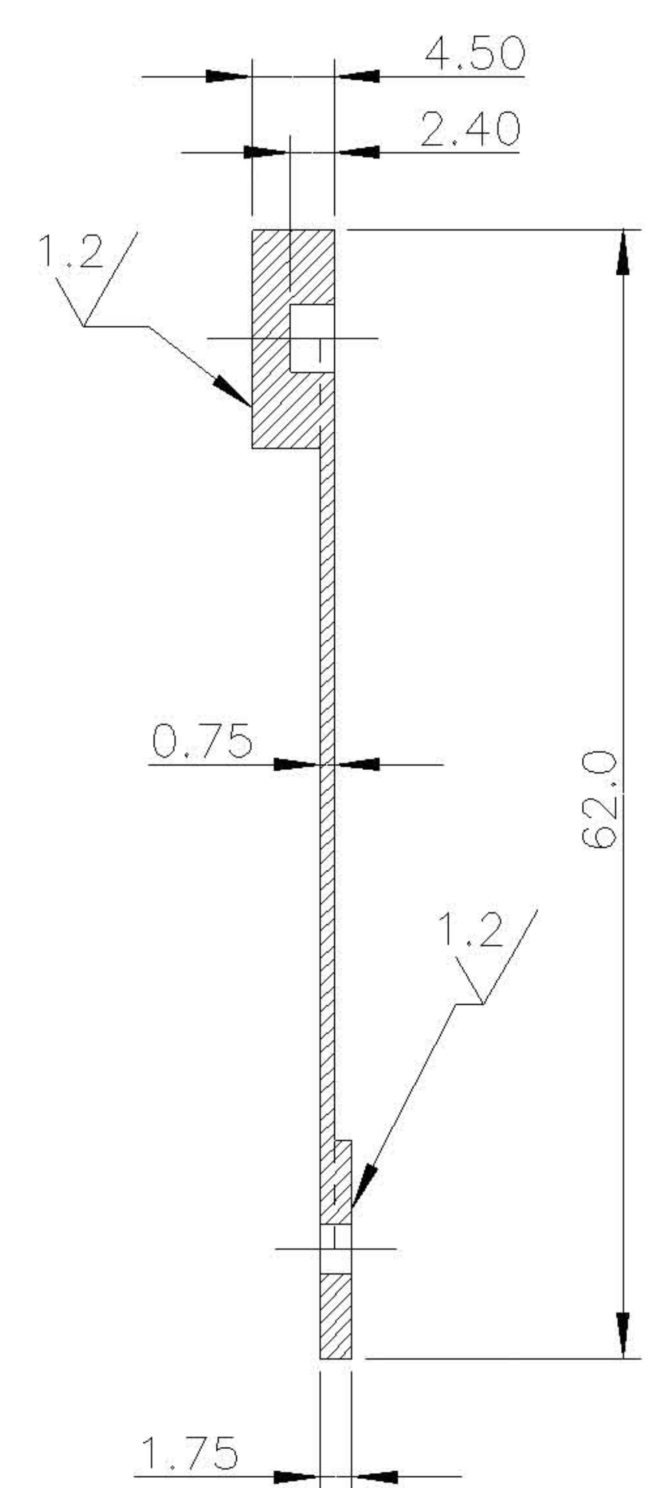
SECTION A-A
