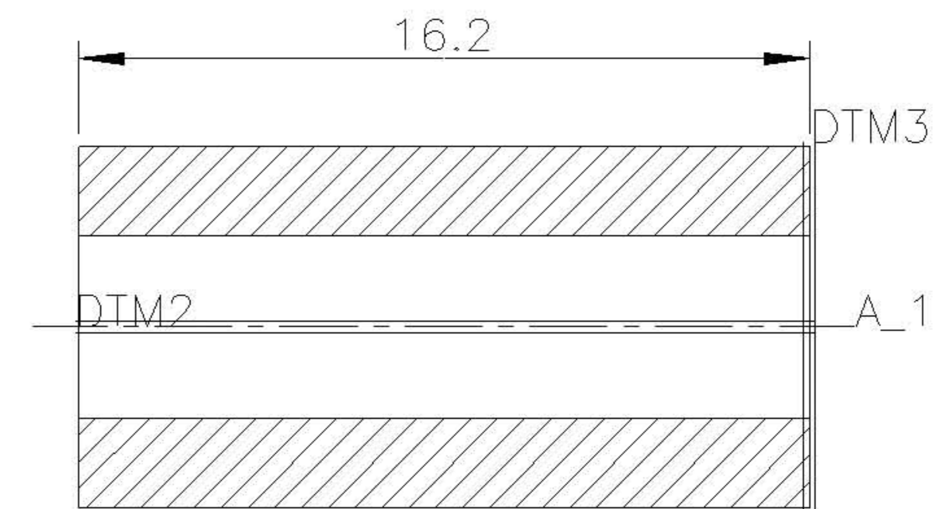
SECTION A-A
