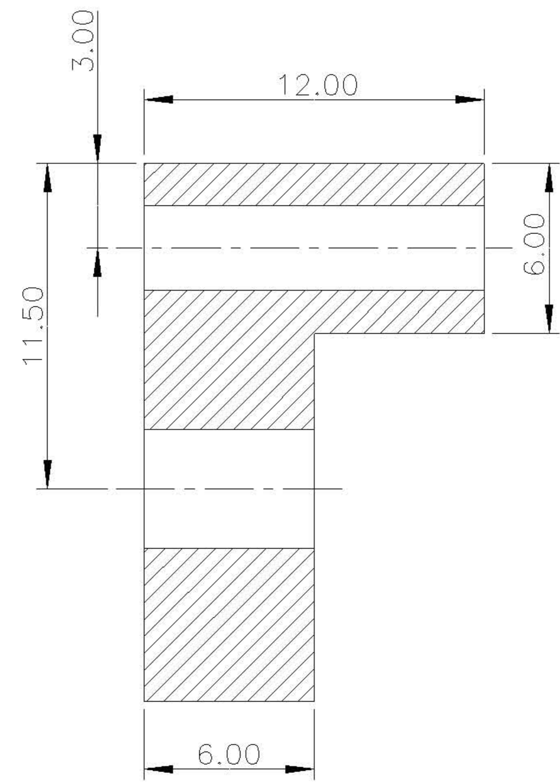
SECTION A-A
